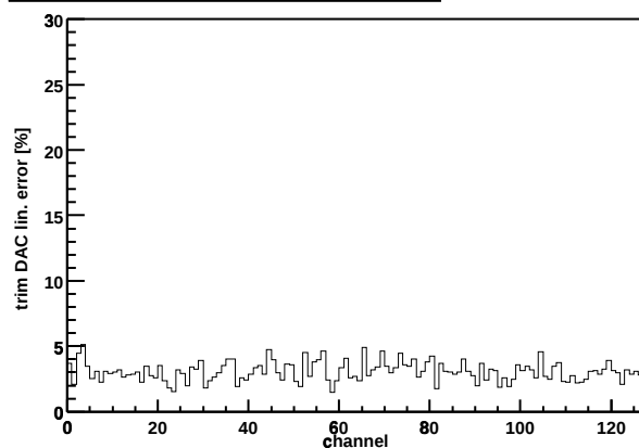
Chip Z36459A-W03-X04-Y09 trim DAC lin. error
