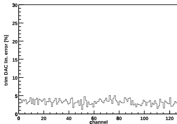
Chip Z36459A-W03-X06-Y09 trim DAC lin. error
