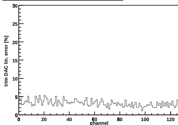
Chip Z36459A-W03-X07-Y09 trim DAC lin. error
