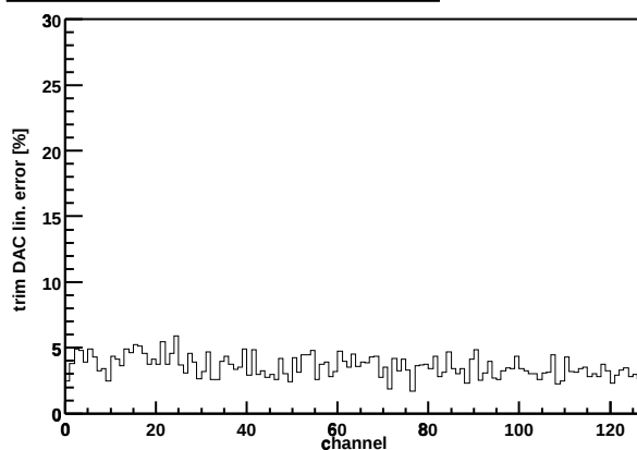
Chip Z36459A-W03-X10-Y09 trim DAC lin. error
