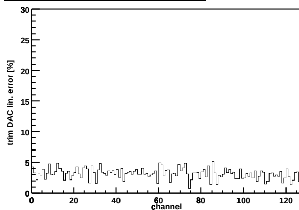
Chip Z36459A-W03-X11-Y09 trim DAC lin. error
