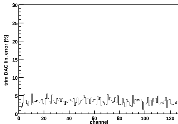
Chip Z36459A-W04-X05-Y01 trim DAC lin. error
