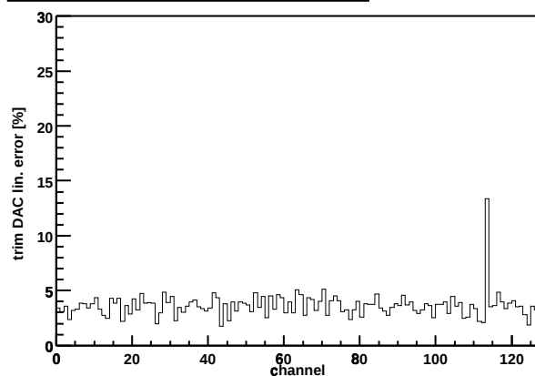
Chip Z36459A-W04-X06-Y06 trim DAC lin. error
