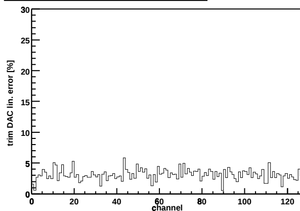
Chip Z36459A-W04-X06-Y09 trim DAC lin. error
