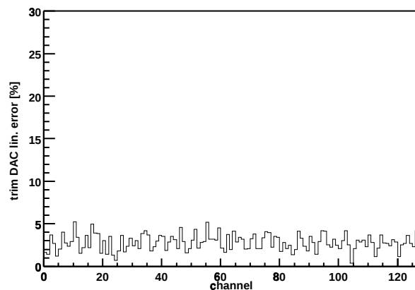
Chip Z36459A-W04-X06-Y10 trim DAC lin. error
