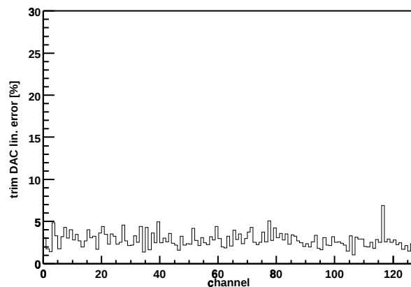
Chip Z36459A-W04-X06-Y13 trim DAC lin. error
