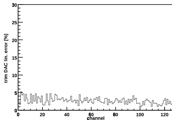
Chip Z36459A-W04-X07-Y06 trim DAC lin. error
