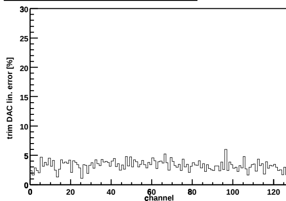
Chip Z36459A-W04-X07-Y07 trim DAC lin. error
