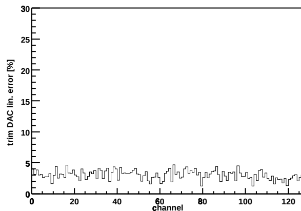
Chip Z36459A-W04-X07-Y08 trim DAC lin. error
