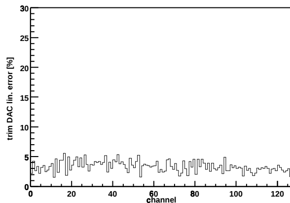
Chip Z36459A-W04-X12-Y09 trim DAC lin. error
