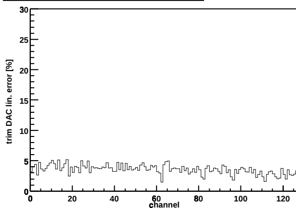
Chip Z36459A-W04-X16-Y09 trim DAC lin. error
