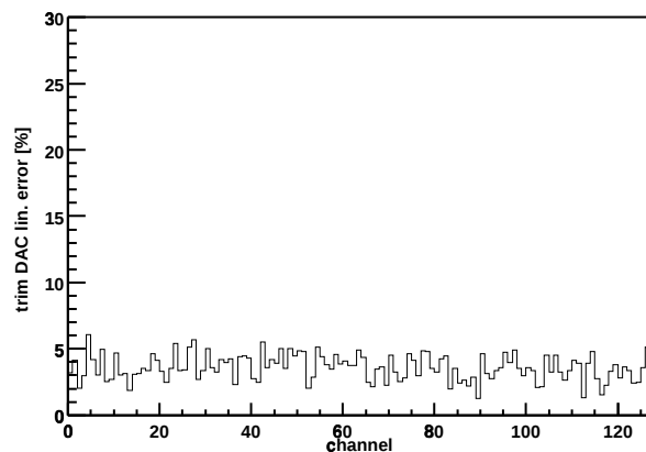
Chip Z36459A-W06-X10-Y09 trim DAC lin. error
