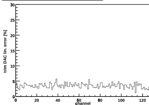
Chip Z36459A-W06-X12-Y09 trim DAC lin. error
