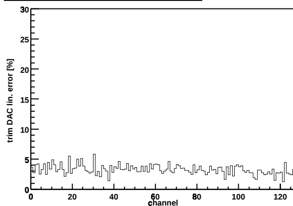
Chip Z36459A-W06-X14-Y09 trim DAC lin. error
