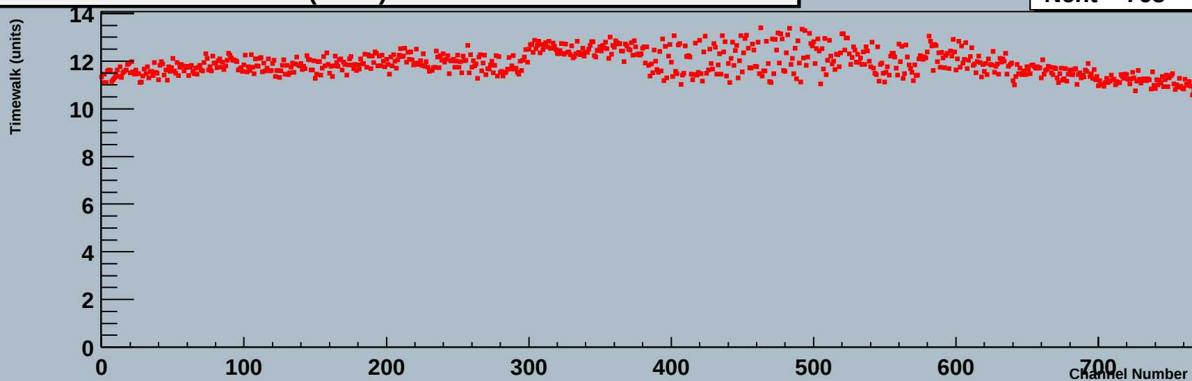
Timewalk (nS) module 3 link 1
