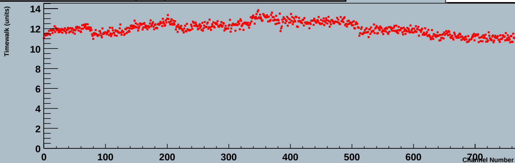
Timewalk (nS) module 3 link 0
