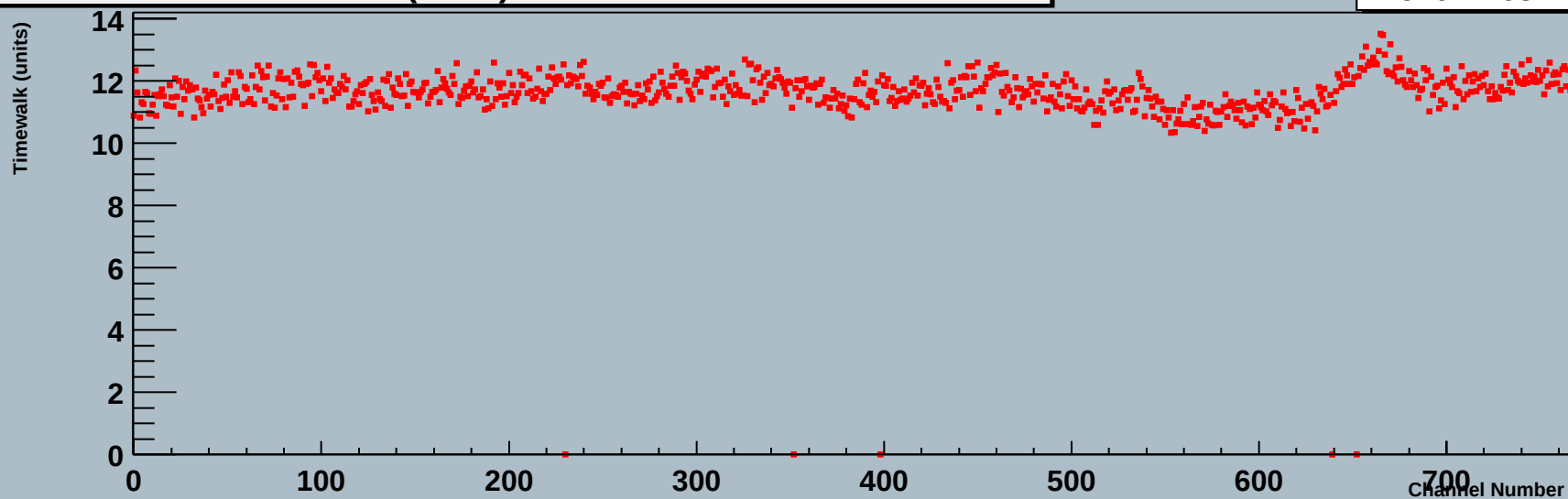
Timewalk (nS) module 1 link 0
