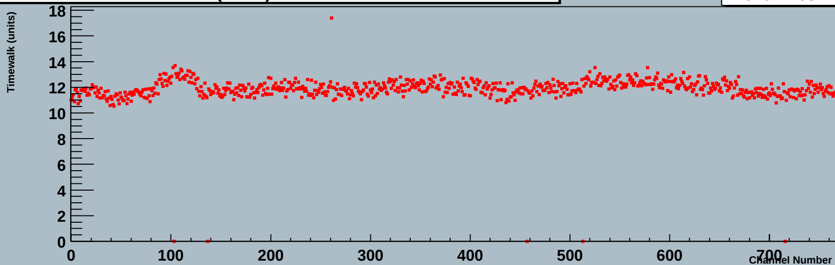
Timewalk (nS) module 1 link 1
