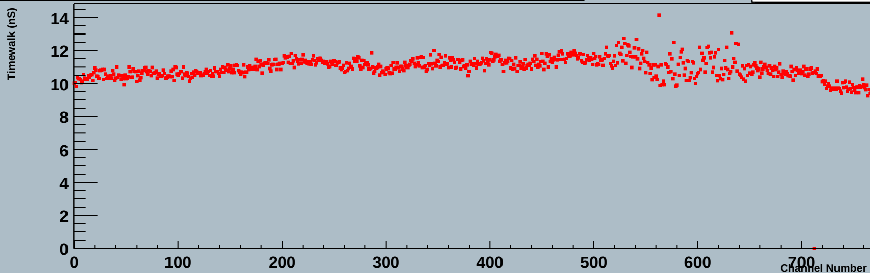
Timewalk (nS) module 5 link 1
