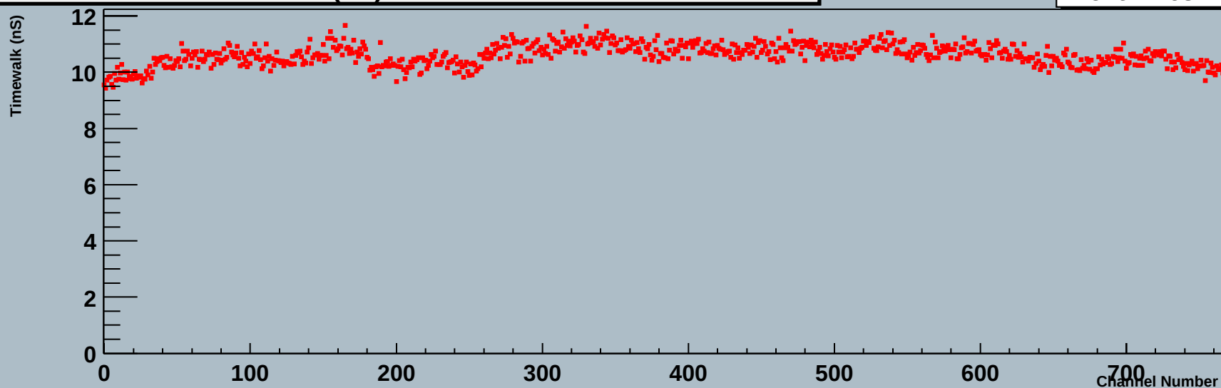
Timewalk (nS) module 5 link 0
