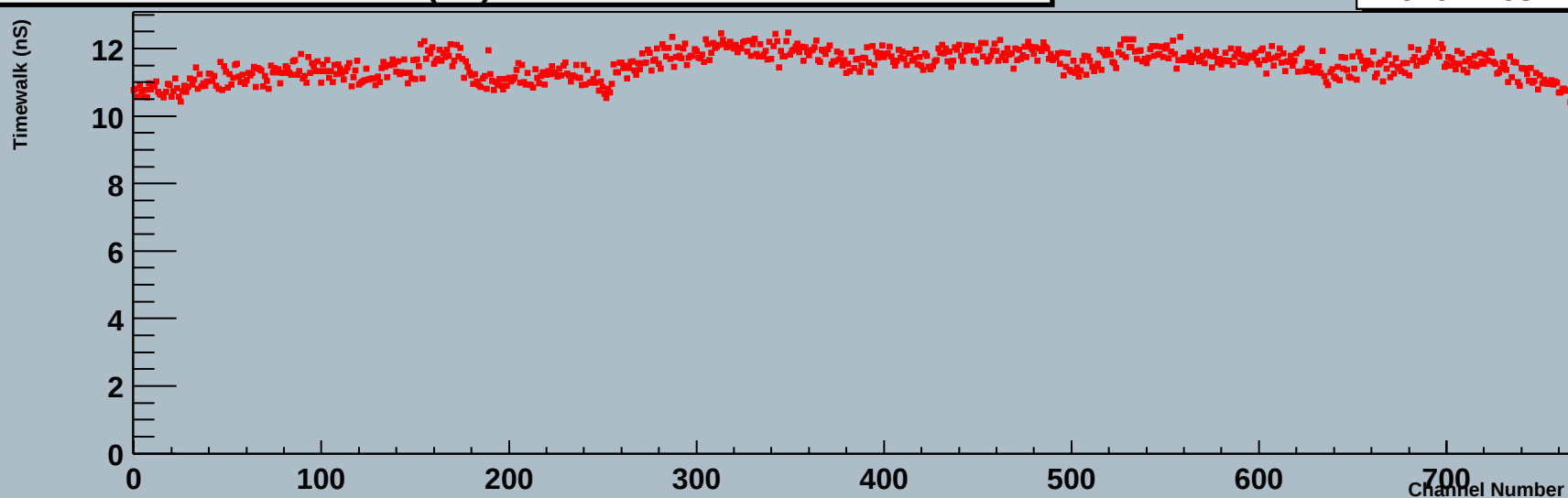
Timewalk (nS) module 0 link 0
