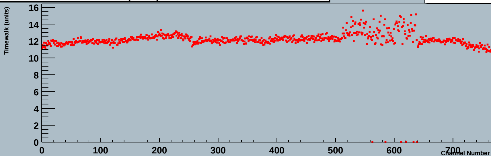
Timewalk (nS) module 0 link 1
