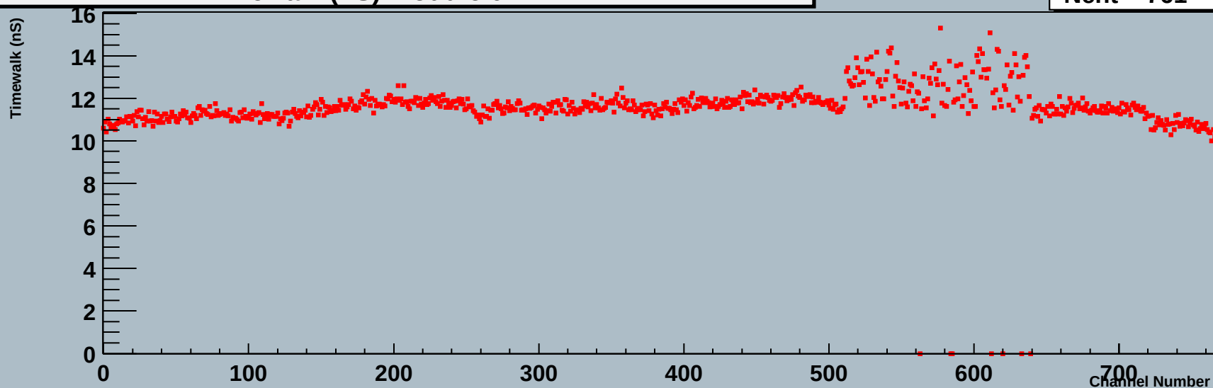
Timewalk (nS) module 0 link 1
